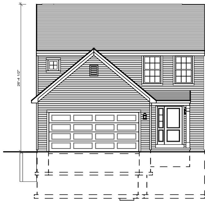
AZALEA SCALE: 3/32" = 1'-0"
